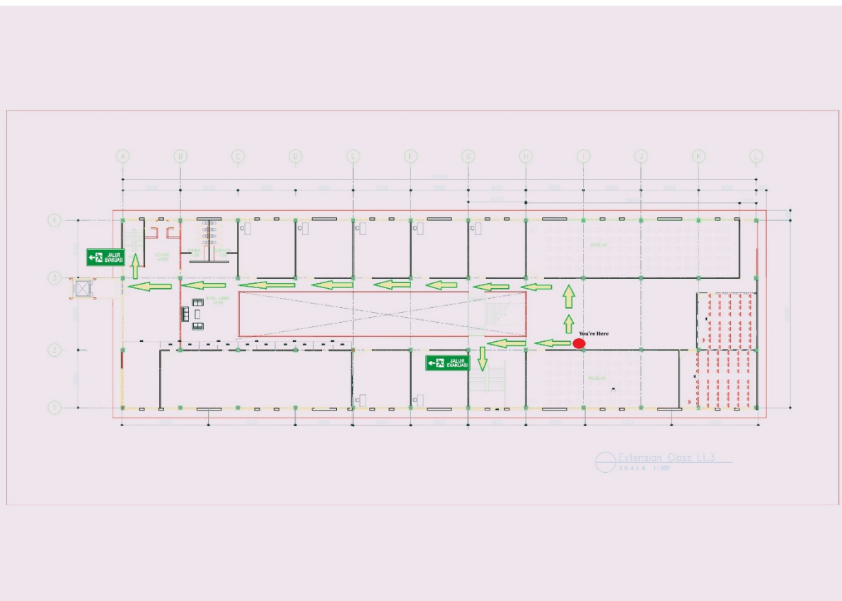
Gambar. Jalur Evakuasi lt. 3
