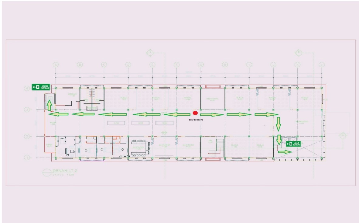
Gambar. Jalur Evakuasi lt. 3
